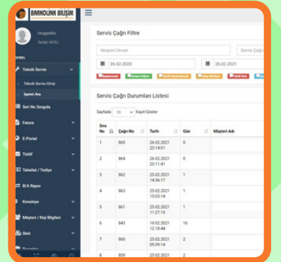
CRM YAZILIMI
